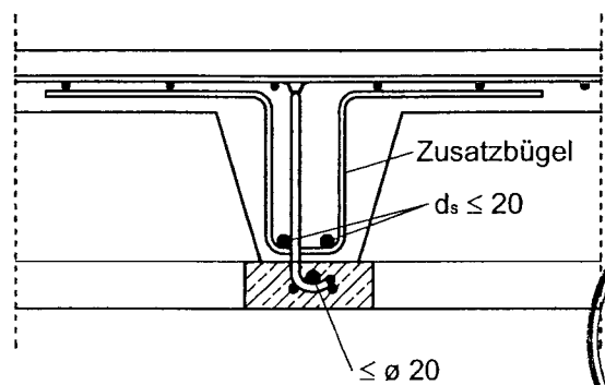
Bild 10: Rippelementdecke und Elementrippendecke mit Zusatzbewehrung
