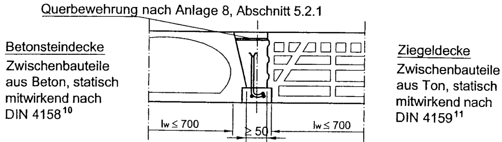
Bild 6: Rippendecke nach Anlage 8, Abschnitt 5
