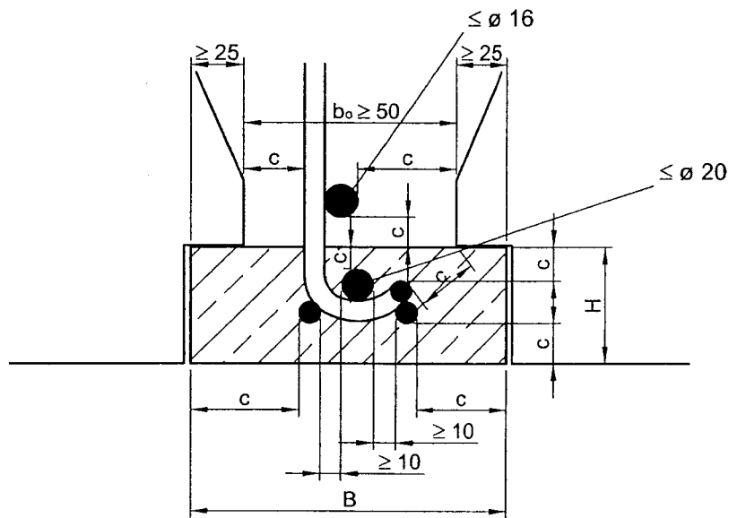
Bild 11: Betonfußleiste mit S-Träger und Zusatzbewehrung
